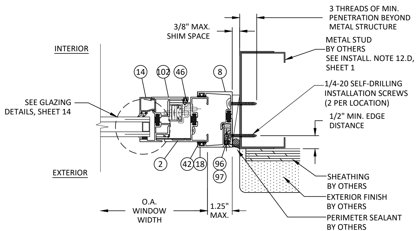
C 6 HORIZONTAL SECTION VENT JAMB - METAL STUD FRAME EXT. SET RECEPTOR - TYP. - INSWING
