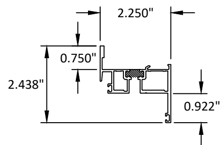
102 VENT - INSWING
