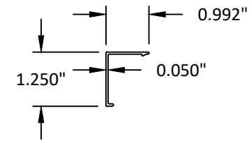
66 1 1/4\"/>
